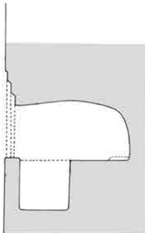
نما و طرح مقطع عمودی استودان شماره ۱، سنگ چله گاه
